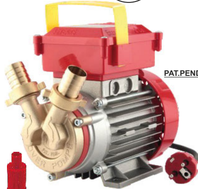
ROVER 25 CE
