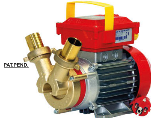
ROVER 30 CE
