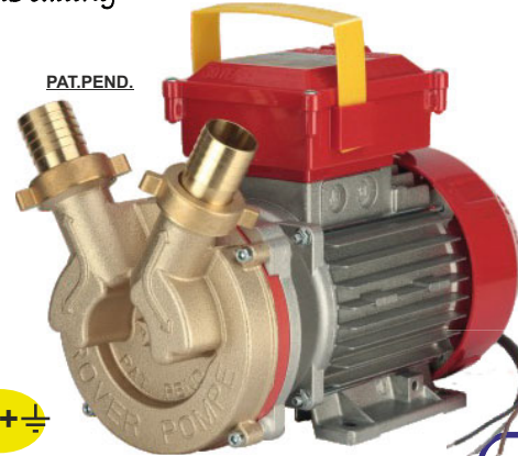
BE-T 40
