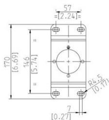
Piastra fissaggio a pavimento
